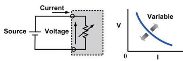
CP Mode
